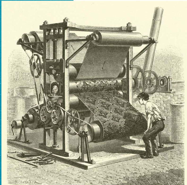
FIG. 303. — Machine à gaufrer le velours d'Utrecht.
